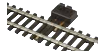
55270 Anschluss-Clip 7,45 €* Anschluss-Clip mit EMV-Entstörelement. Passend zu G231
